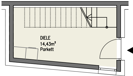
ERDGESCHOSS EINGANGSGESCHOSS
